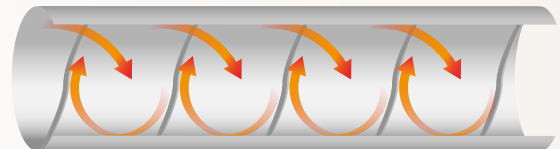
Tubi con anelli elicoidali Babcock Wanson
